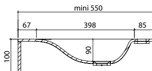
COUPÉ
